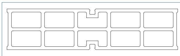
Versteving van het rooster met nominale breedte 100 (500 x 123 mm)
