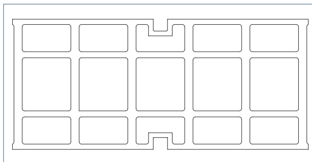
Versteving van het rooster met nominale breedte 200 (500 x 223 mm)
